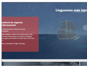
ReactJS web
